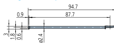
12AAE898 (2µm)* 12AAE914 (5µm)** ( ) : Tip radius *Tip angle: 60° **Tip angle: 90°
